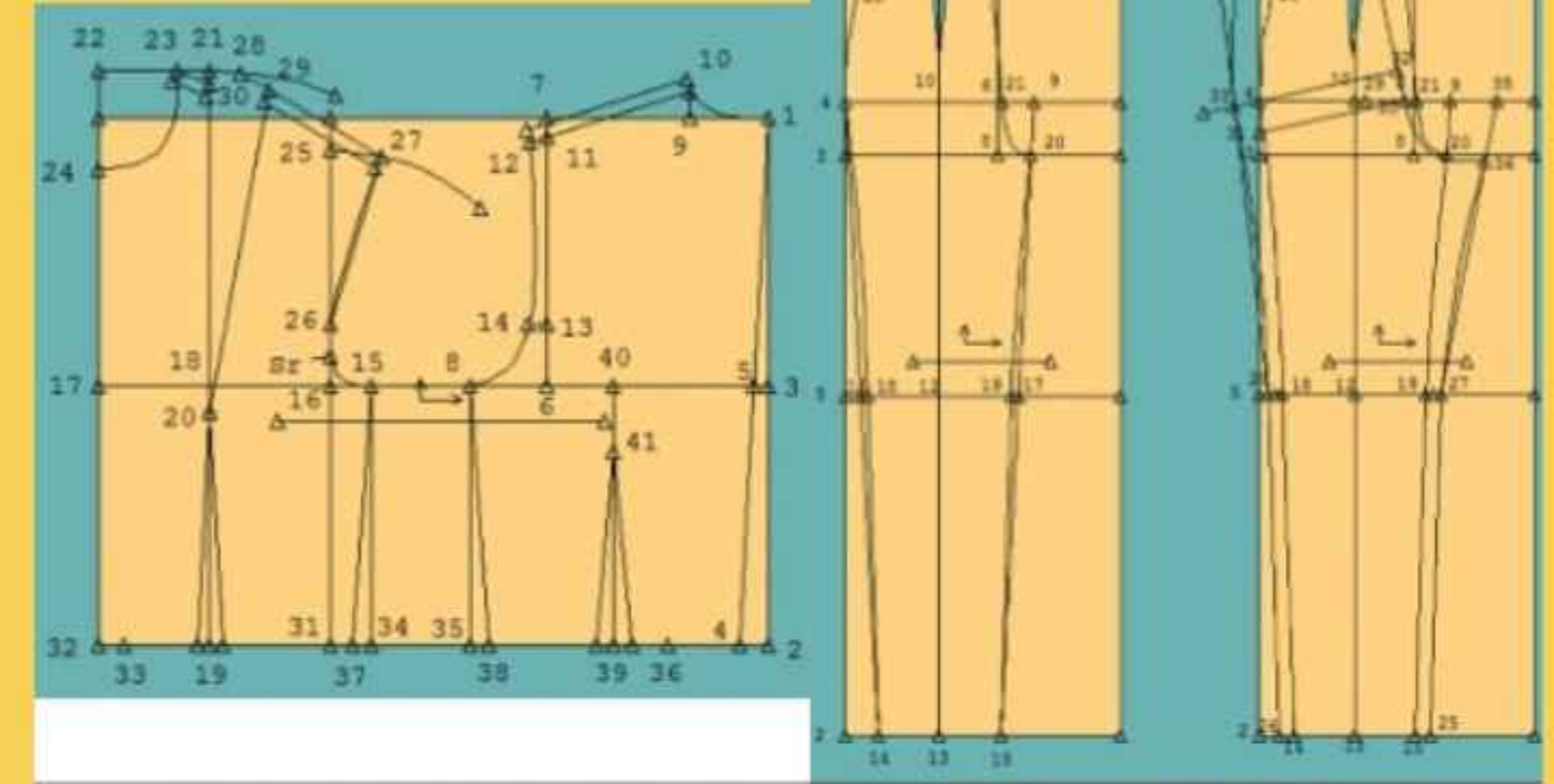
Основна конструкција блузе
